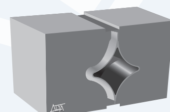
Açılı Tam Yıldız Zımba Tapered Full Star Punch 40/37x22x23.7mm
